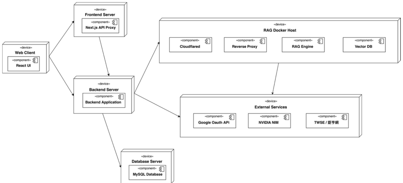
▲圖 7-1-1 佈署圖
