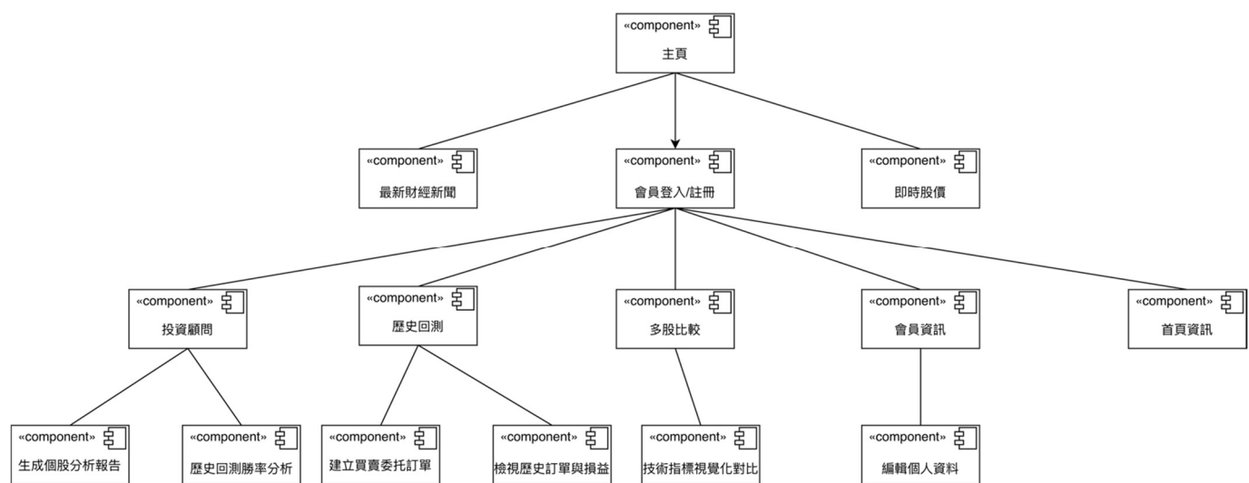
▲圖 7-3-1 元件圖
