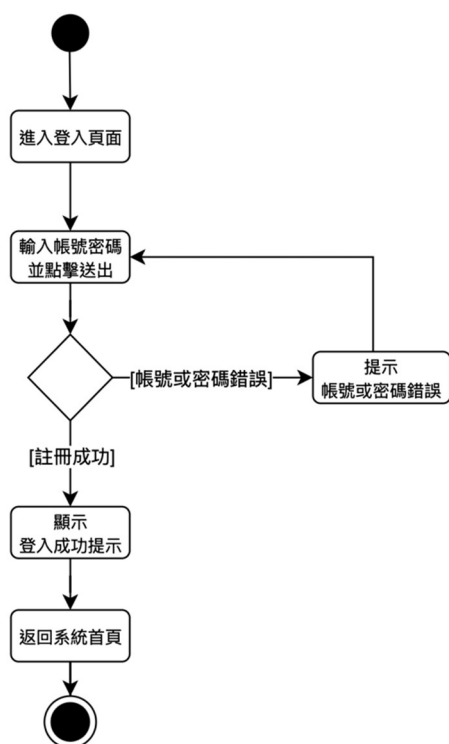
▲圖 5-3-2 會員登入之活動圖
