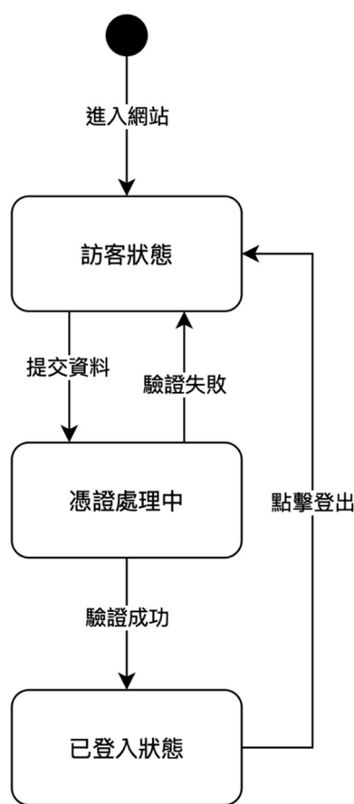
▲圖 7-4-1 會員登入/註冊之狀態機圖
