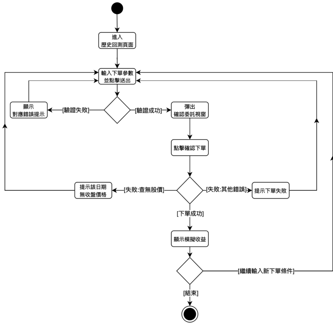
▲圖 5-3-6 歷史回測之活動圖
